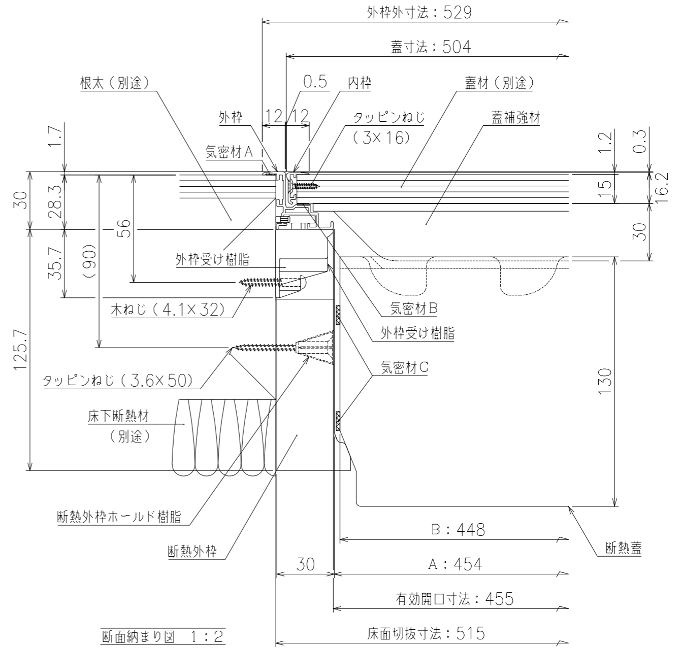
HXD350型 規格寸法 (単位: mm)
